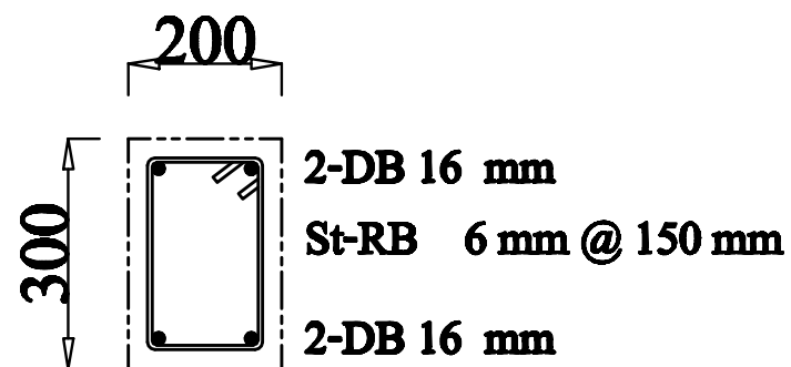
ขยาย B2
