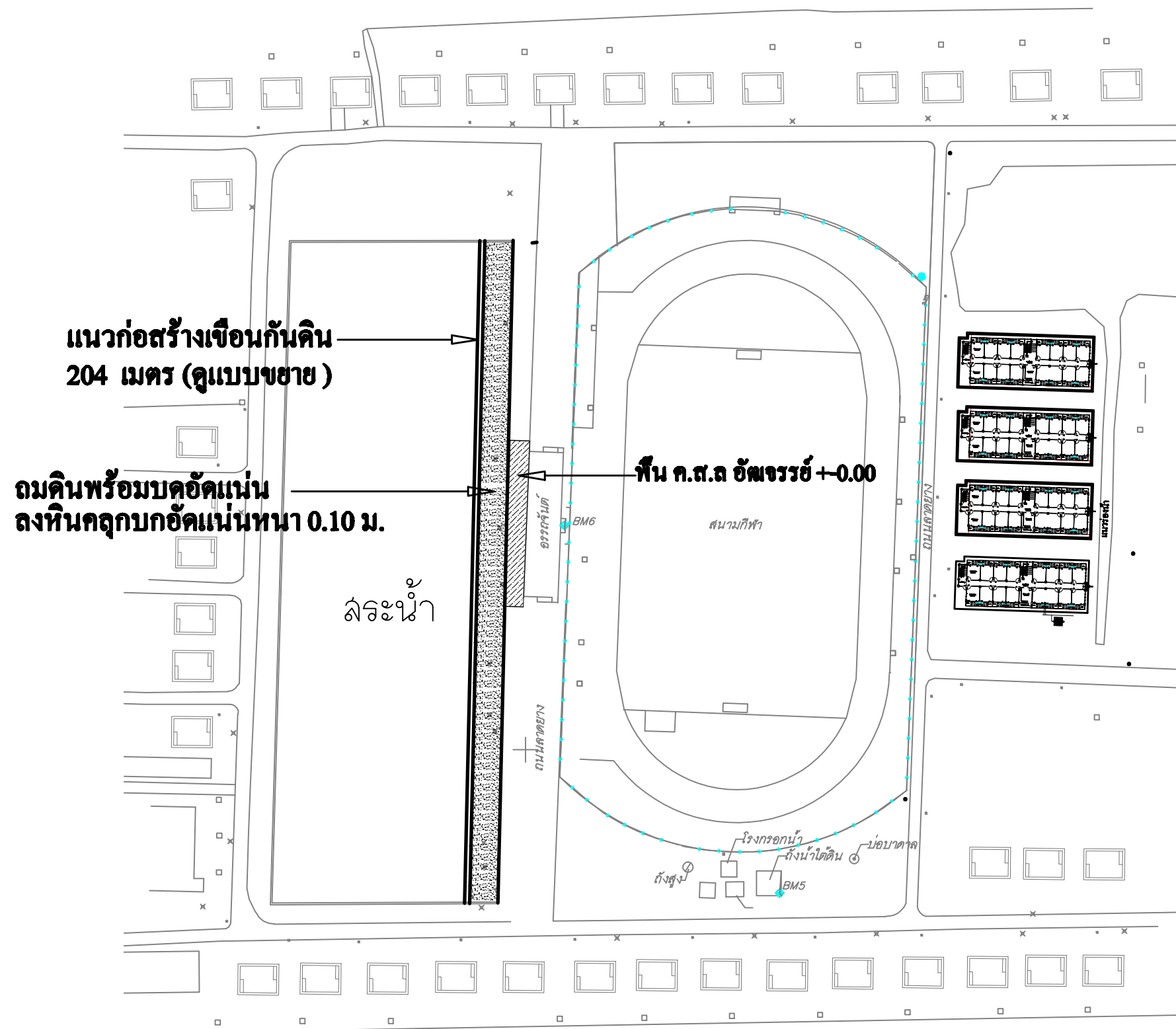
แบบผังบริเวณเขื่อนกันดิน
