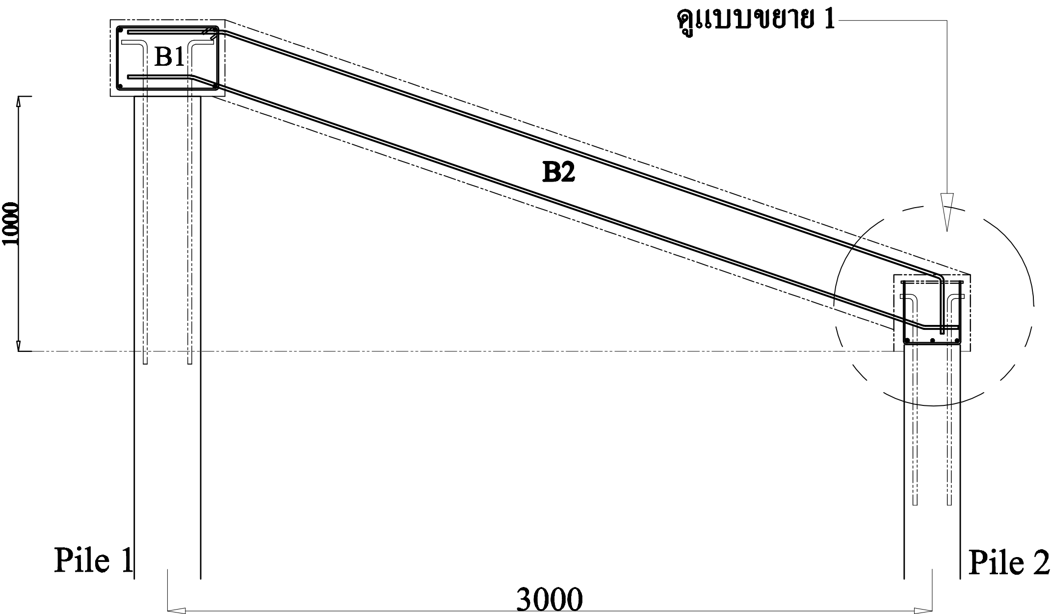
แบบขยายคานยึดกับหัวเสา
