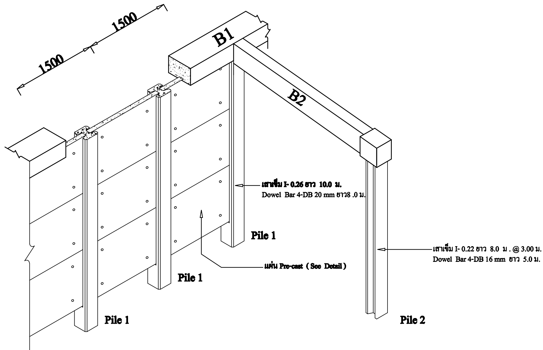
รูปแบบ 3 มิติ
